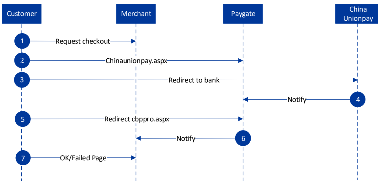
China UnionPay Prozessablauf
