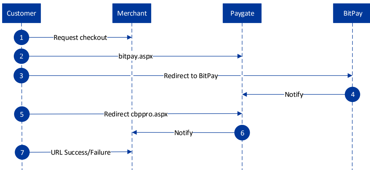
BitPay Prozessablauf
